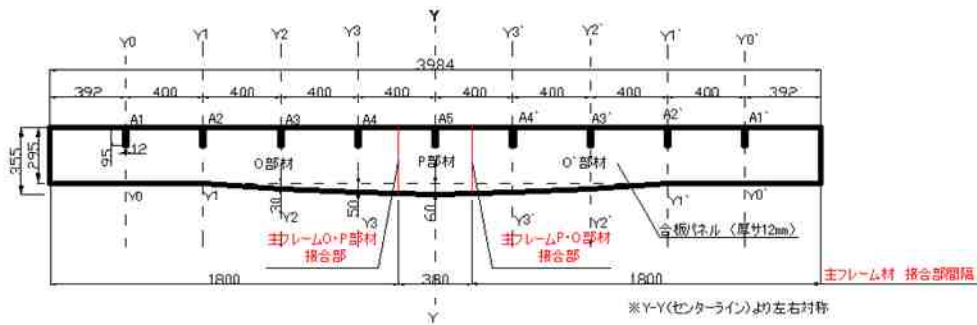
型枠部材 主フレーム部 側面図
