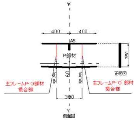
型枠部材 主フレーム部 P部材
