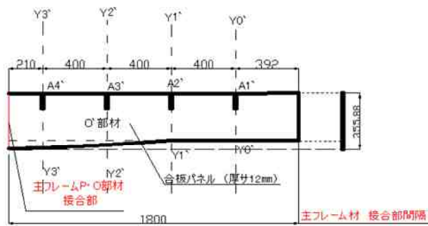
型枠部材 主フレーム部 O'部材
