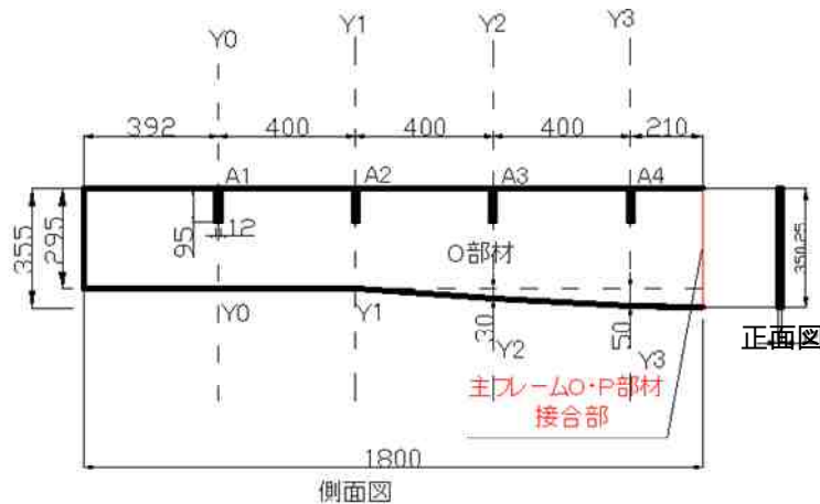
型枠部材 主フレーム部 O部材
