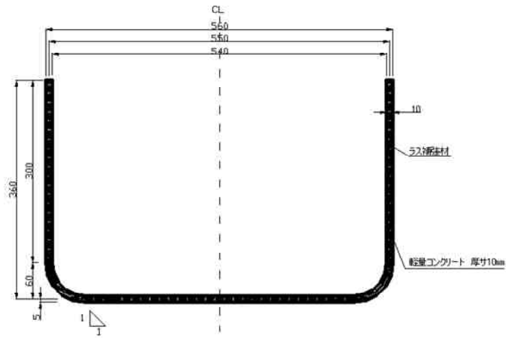
Y4-Y4詳細断面図
