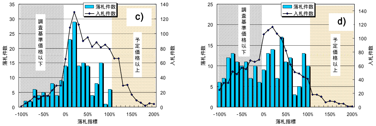
図 - 6 工事種別毎における落札指標の頻度分布, a) 全工種, b) 一般土木, c) PC, d) 鋼橋上部工
