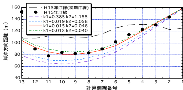
図－8 数値計算による汀線変化の再現
