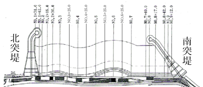
図-3 人工海岸の平面図と測線位置図
