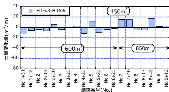
図－7 土量変化量 (H16年－H15年)
