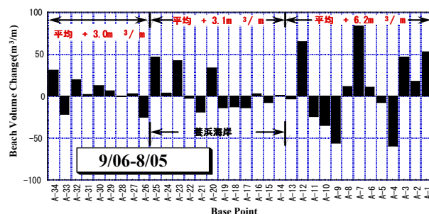
図-6 1年間の土量変化
