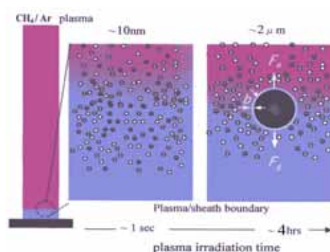
図3 MSCP の成長メカニズム
