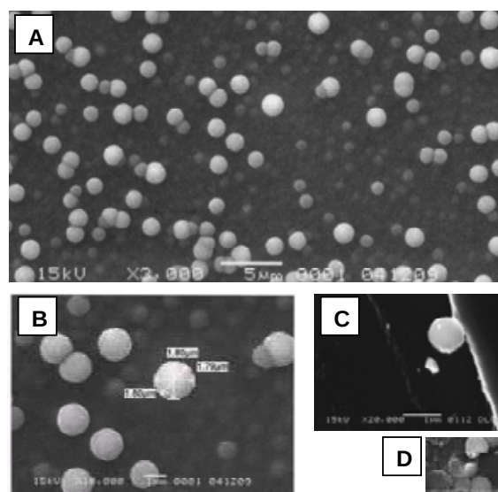
図2 A: 初めて見出した球状粒子のSEM像, B: 真球度の測定, C: ダイヤモンド針によるスクラッチで分った球状(粒子の側面SEM像)。D: 粒子内部
